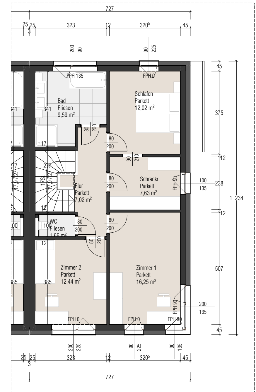
OBERGESCHOSS | 1:100
